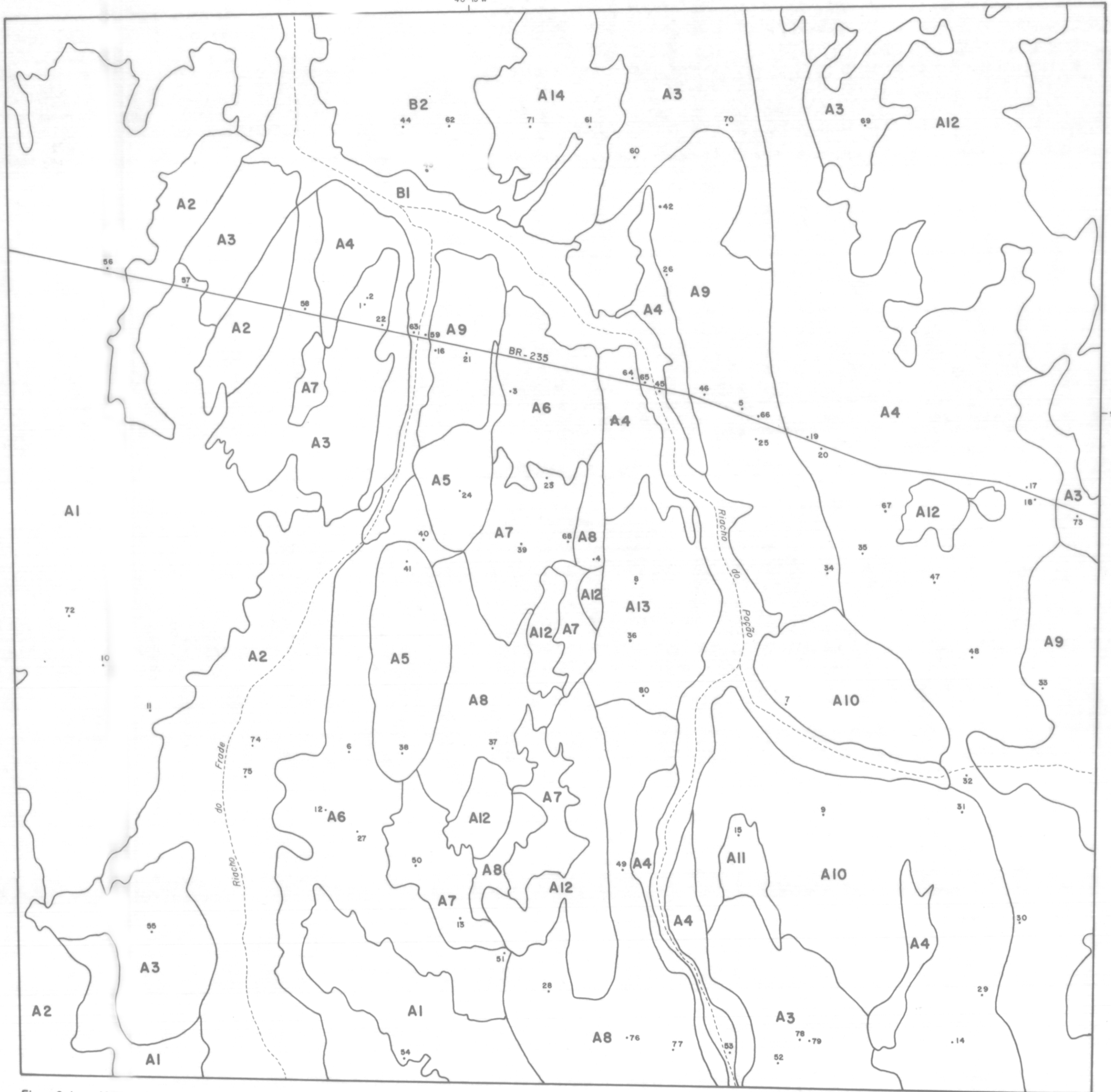
Fig. G.1 - Mapa de unidades geomorfológicas obtido a partir da análise visual das fotografias aéreas.
